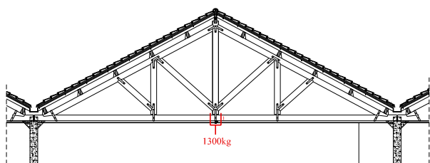
1 APOIO - 1300kg
